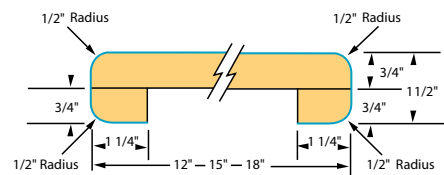
BAR TOP EWB-12 EWB-15 EWB-18
