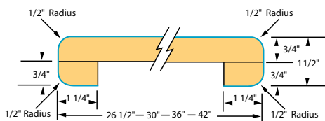
BAR TOP EWB-26 1/2 EWB-30 EWB-36 EWB-42
